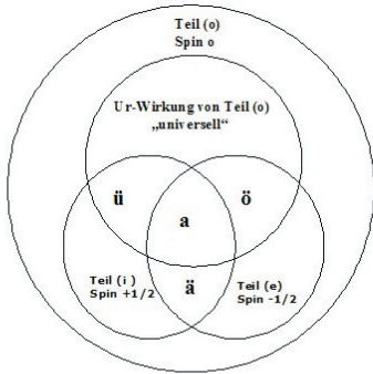
Kategoriale Korrelationen bei entanglement in Figur 2 (Zeilinger in Nature arXiv:0704.2529v1 19.4.2007)
